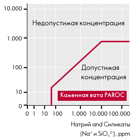
Рис. 4. Состав вымываемых водой ионов, ASTM C 795
