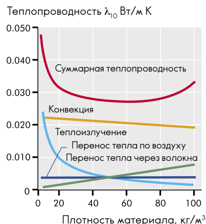
Рис. 1. Теплопроводность каменной ваты
